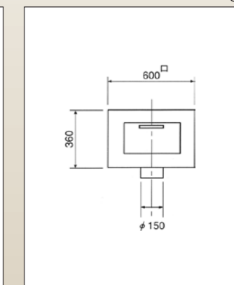
●ユニット図 Unit Drawing
