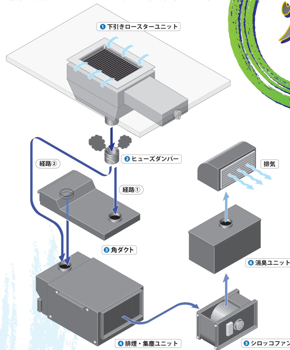
[煌]排煙消臭装置仕様
